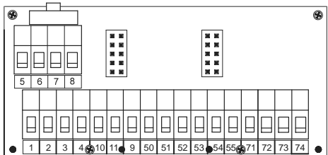
Anschluss 2-Leiter
