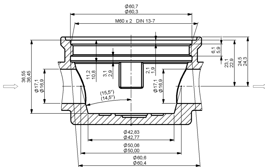
Bild 2 - Schnittstelle „DM1“
